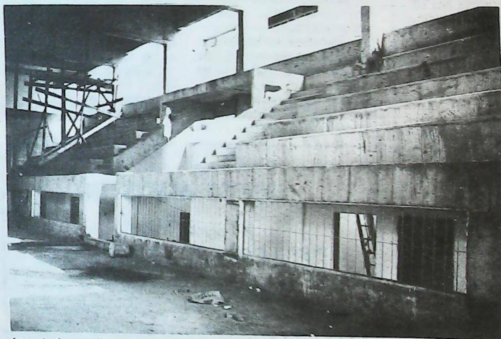
Aspecto das arribancadas e tribuna de honra. Na parte inferior os vestiários.
